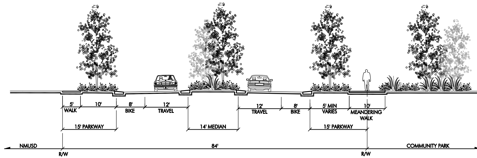
SECTION D-D
